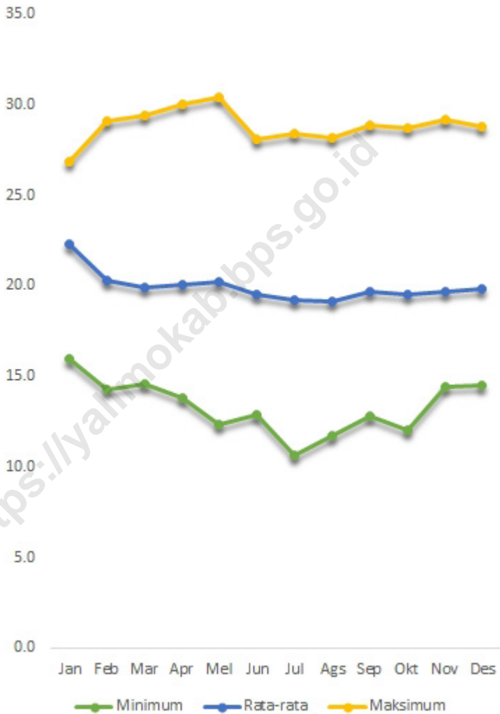
Gambar 1.3 Suhu Udara Kabupaten Yalimo Tahun, 2020 Figures 1.3 Air Temperature of Yalimo Regency, 2020
