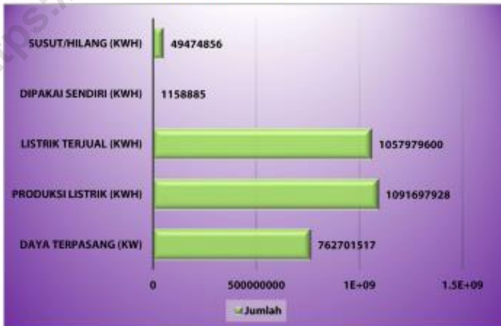
Grafik/Graph 6.2 Daya Terpasang, Produksi dan Distribusi Listrik PT. PLN (Persero) pada Cabang PLN di Kota Yogyakarta, 2020 Installed Power, Production and Distribution of Electricity in Yogyakarta Municipality, 2020
