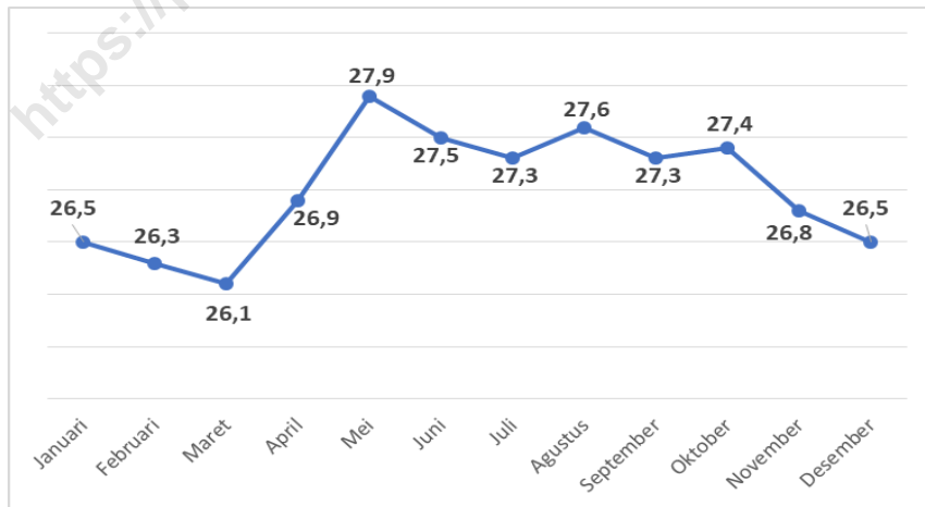
Gambar/Figure 1.2 Rata-rata Suhu Udara di Kota Pangkalpinang per Bulan, 2018 (°C)
