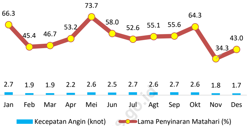
Gambar/Figure 1.5 Lama Penyinaran Matahari dan Kecepatan Angin Menurut Bulan di Kota Jayapura Duration of Sunshine and Wind Velocity by Months in Jayapura City 2018
