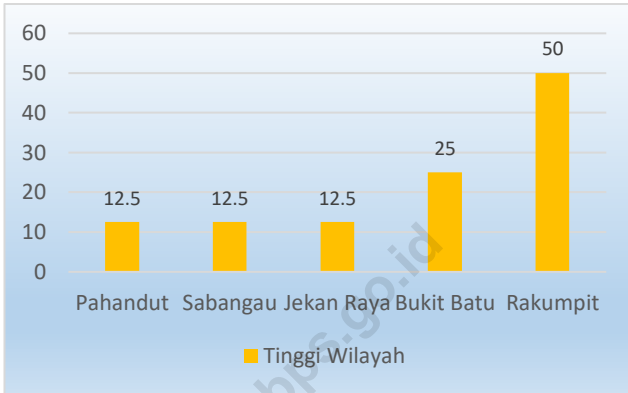
Gambar 1.1 Tinggi Wilayah di Atas Permukaan Laut (DPL) Menurut Kecamatan di Kota Palangka Raya, 2018 Figure High Above Mean Sea Level (AMSL) by Subdistrict in Palangka Raya Municipality, 2018
