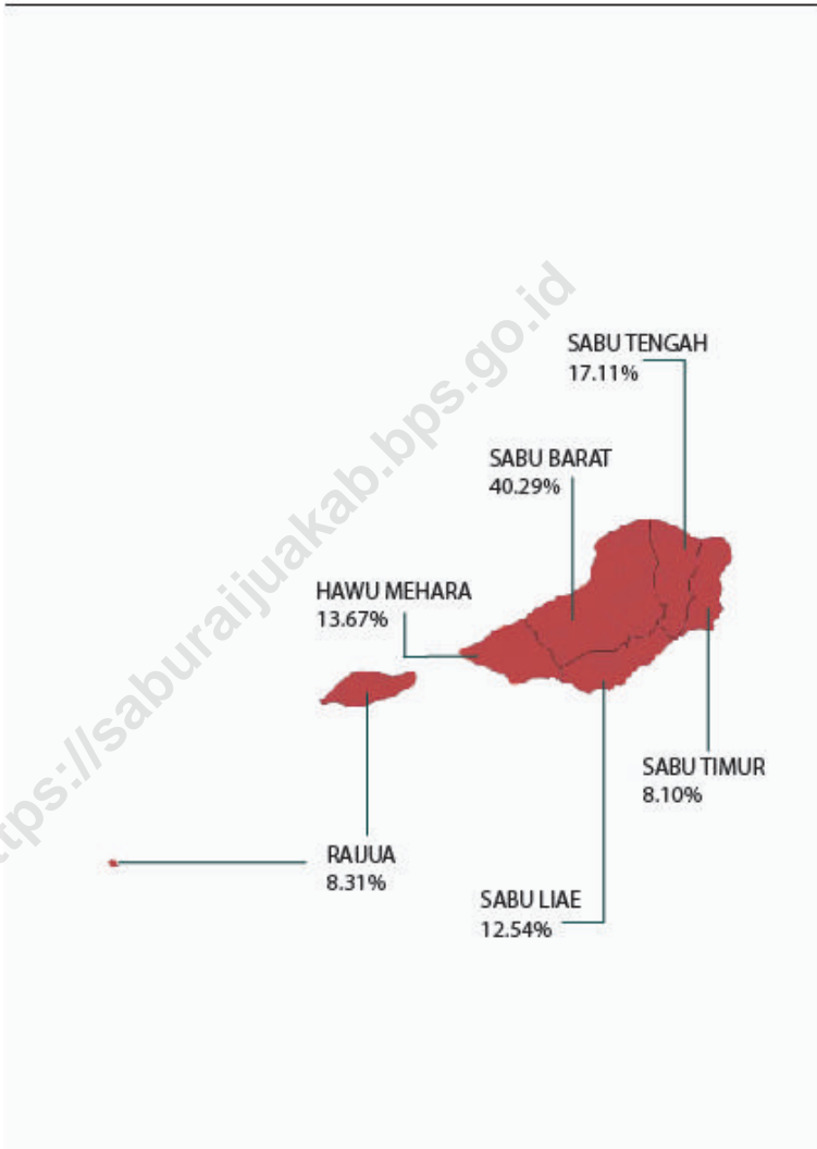
Gambar 13.1 Luas Daerah menurut Kecamatan (%), 2019 Figures 13.1 Area of Subdistrict (%), 2019
