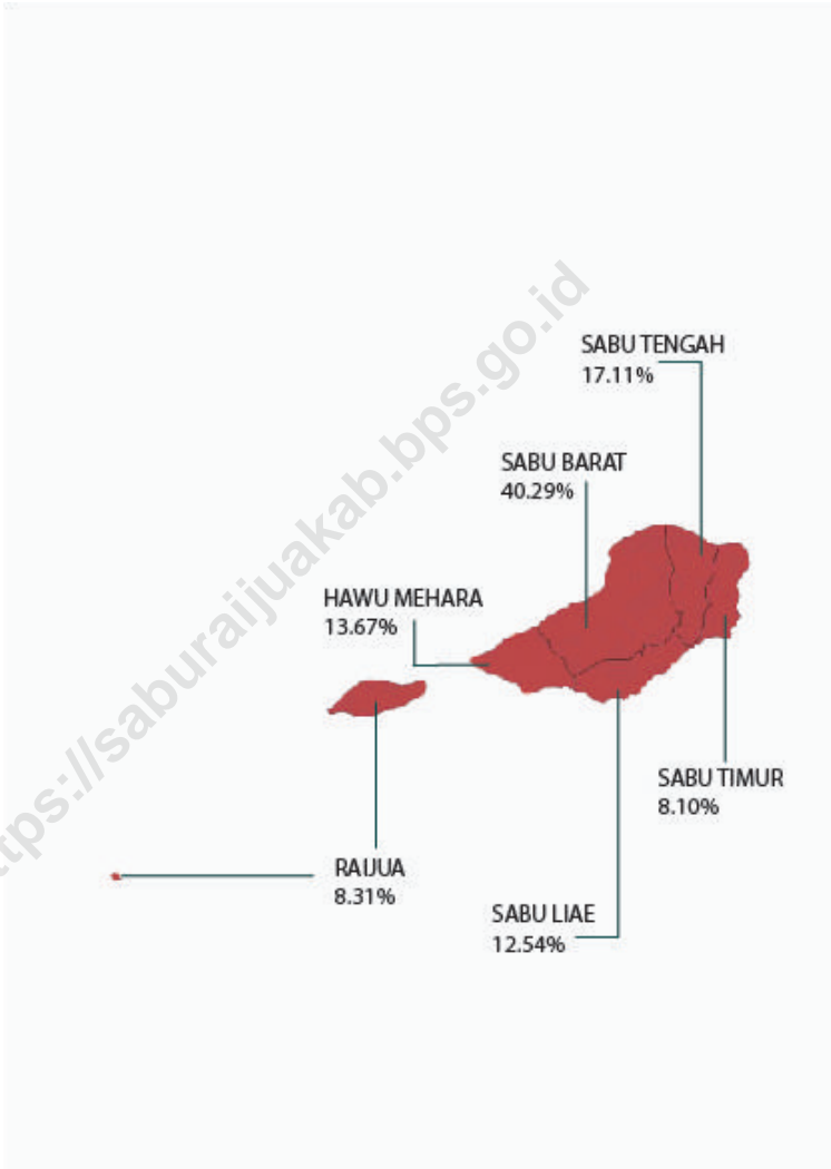
Gambar 3.1 Luas Daerah menurut Kecamatan (%), 2019 Figures 3.1 Area of Subdistrict (%), 2019
