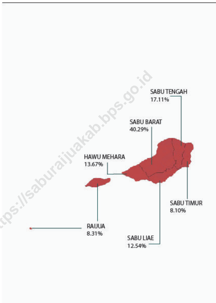
Gambar 8.1 Luas Daerah menurut Kecamatan (%), 2019 Figures 8.1 Area of Subdistrict (%), 2019
