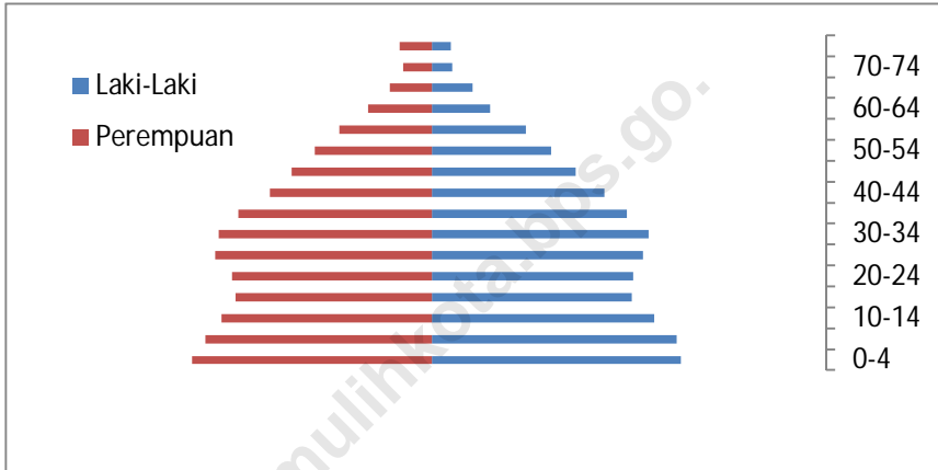
Gambar 5 Piramida Penduduk Kota Prabumulih, 2017 Picture Pyramid Population of Prabumulih Municipality, 2017
