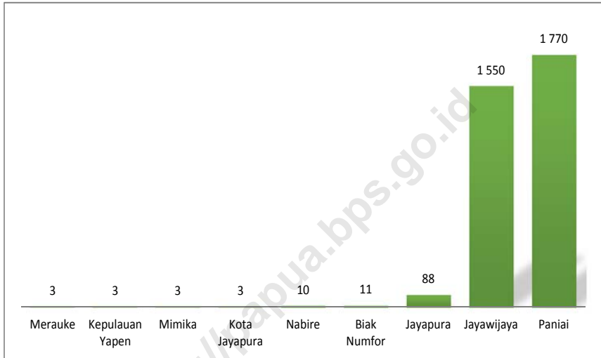
Gambar 1.2. Tinggi Wilayah di Atas Permukaan Laut (DPL) Beberapa Kabupaten/ Kota di Provinsi Papua (meter), 2017 Picture Height Above Mean Sea Level (AMSL) of Some Regency/City in Papua Province (meter), 2017
